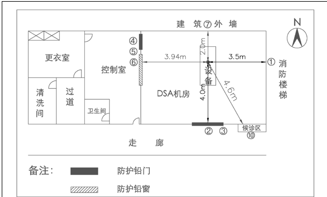
图 11-1 DSA 机房计算点位示意图
