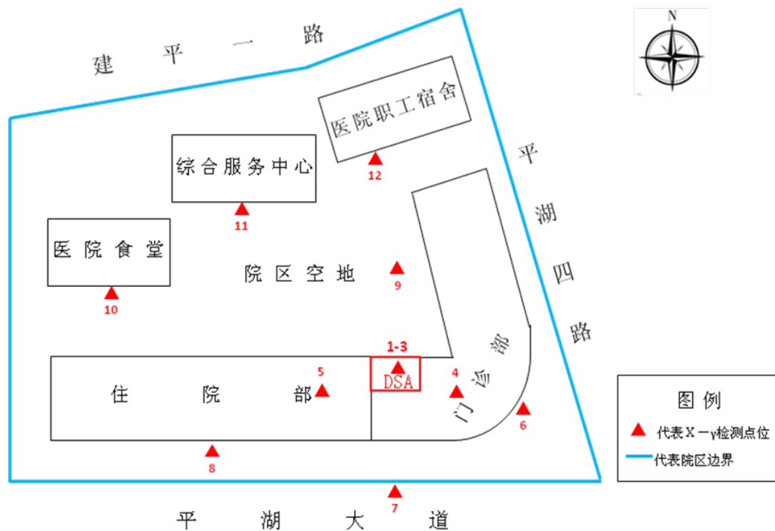
图 8-1 门诊部 DSA 机房周围 X- \gamma 辐射空气吸收剂量率监测点位示意图
